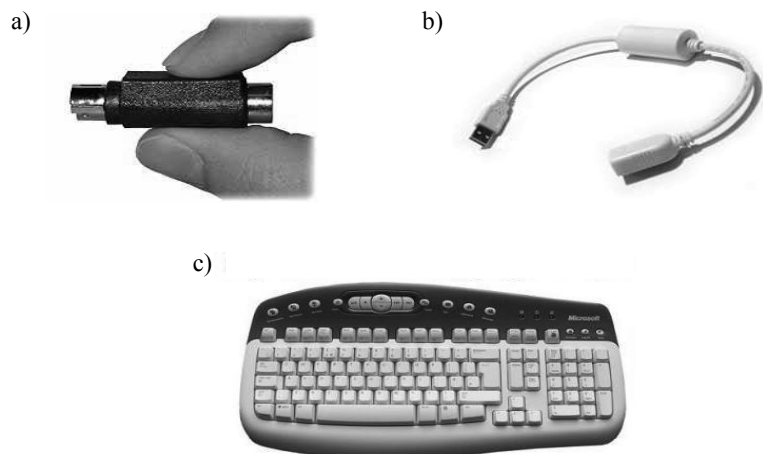
Rys. 5. Urządzenia nazywane keyloggerami, służące do rejestracji wszelkich operacji wykonywanych przy użyciu klawiatury: a) keylogger w postaci „prześciówki” włączanej do gniazda, w które włącza się klawiaturę; b) keylogger w postaci przedłużacza do klawiatury; c) keylogger wbudowany w klawiaturę
